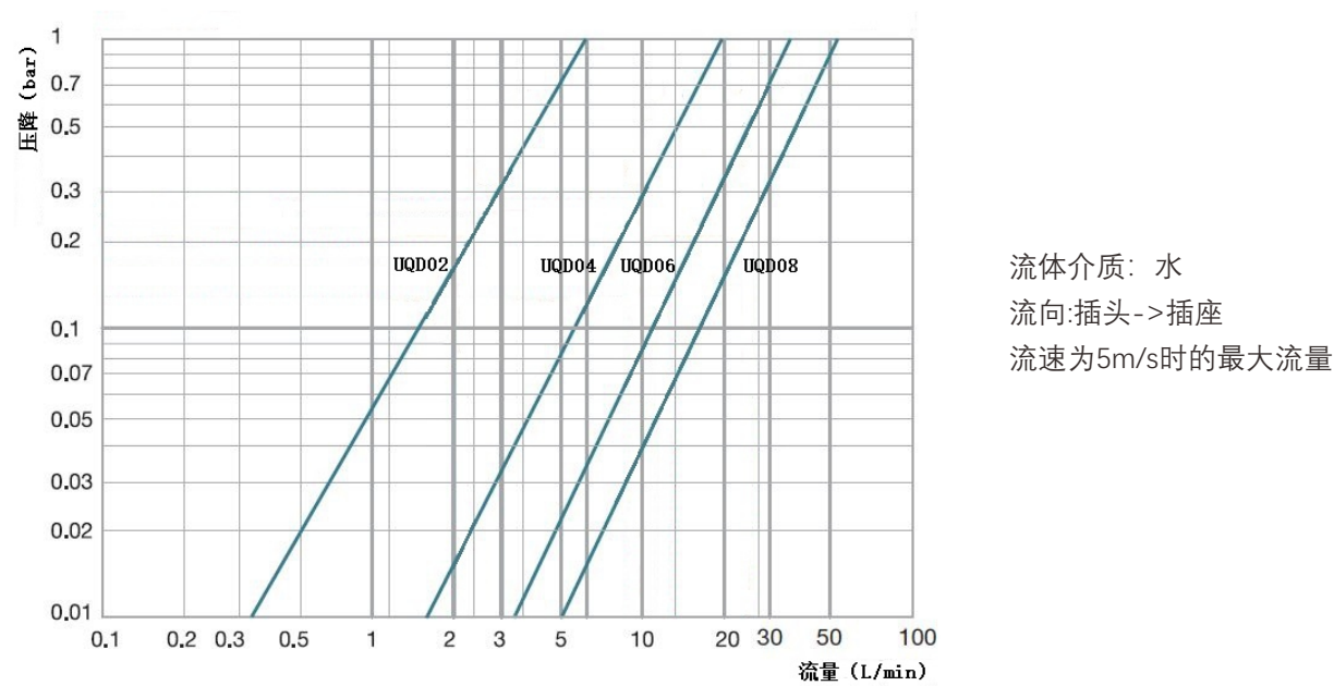
液压流量/压降曲线
