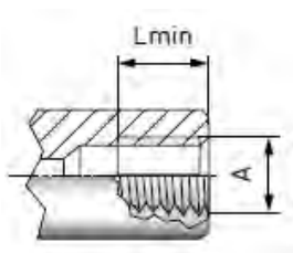
SAE-O形圈凸台密封
