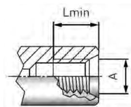
SAE螺纹(根据SAE J1926 / ISO 11926)
