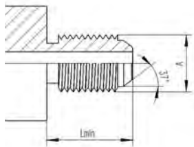
依据SAE J514 JIC37°标准
