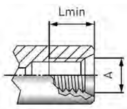
NPT螺纹 (ANSI/ ASME B1.20.1-1983)
