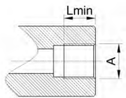
依据公制ISO螺纹
