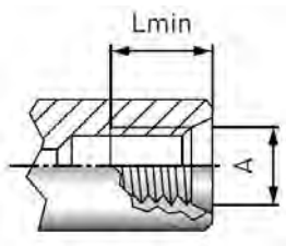
公制 ISO螺纹 (DIN 13 - 根据 ISO 6149-1)
