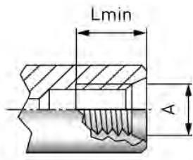
公制ISO螺纹
