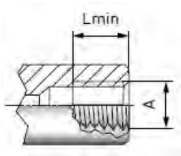
英制直管螺纹 依据DIN ISO228-1
