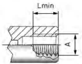
NPT螺纹(依据ANSI/ ASME B1.20.1-1983)
